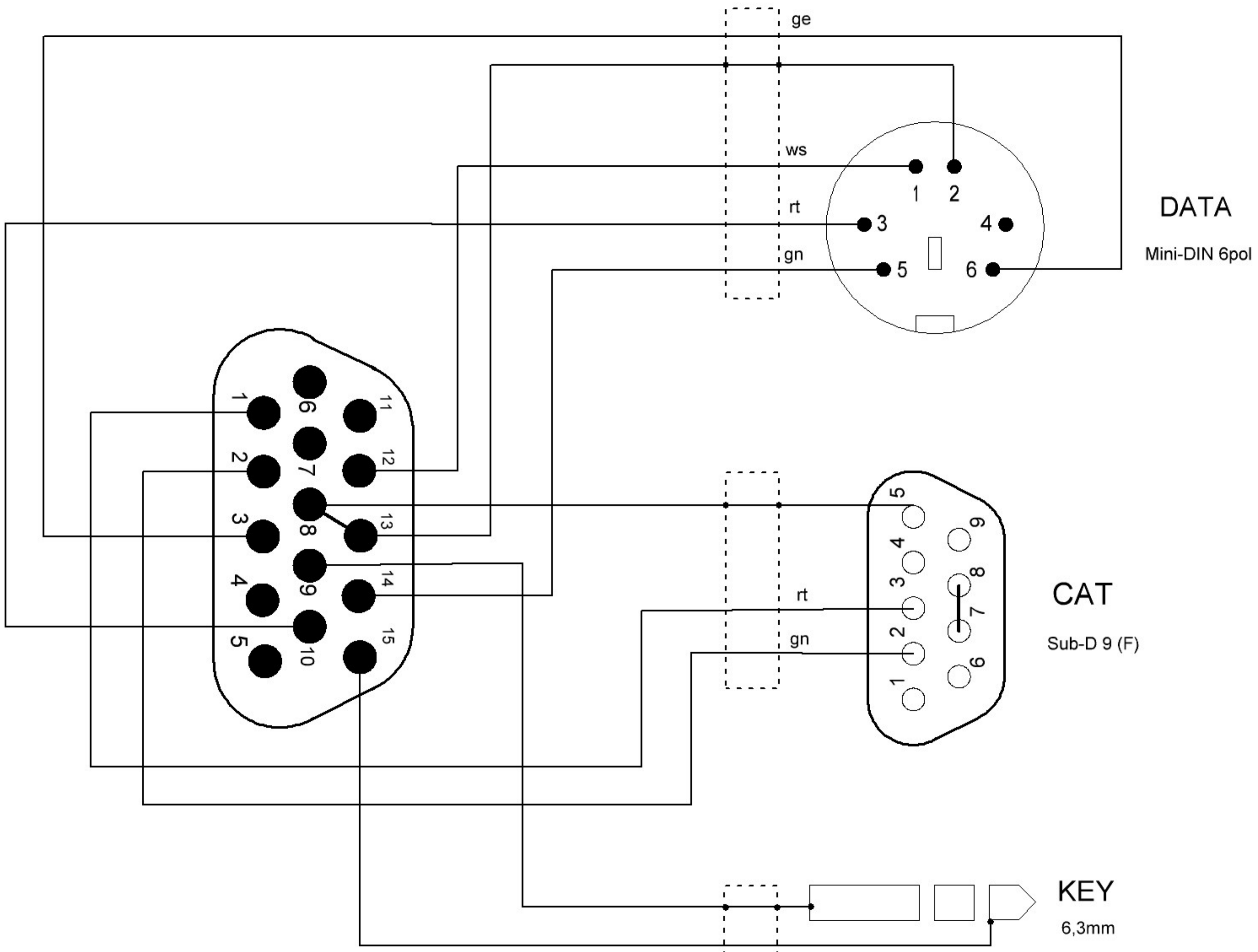
MX22-1 zu FT450 (mit 3,5mm Key-Stecker), FT950, FT1200, FT3000
