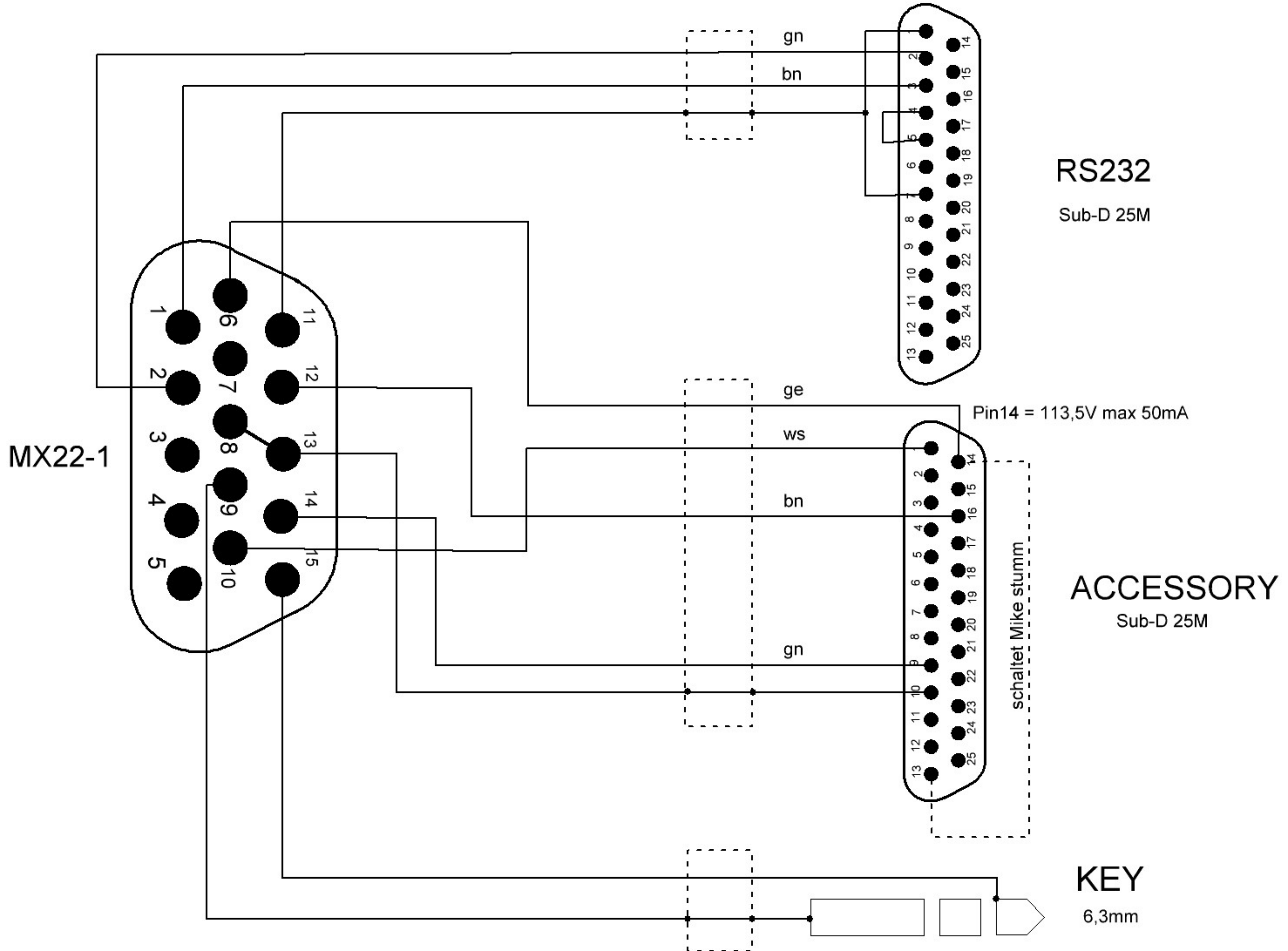
MX22-1 zu JRC JST-145/245
